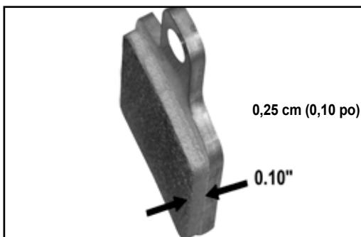
Usure des plaquettes de frein, freins hydrauliques
